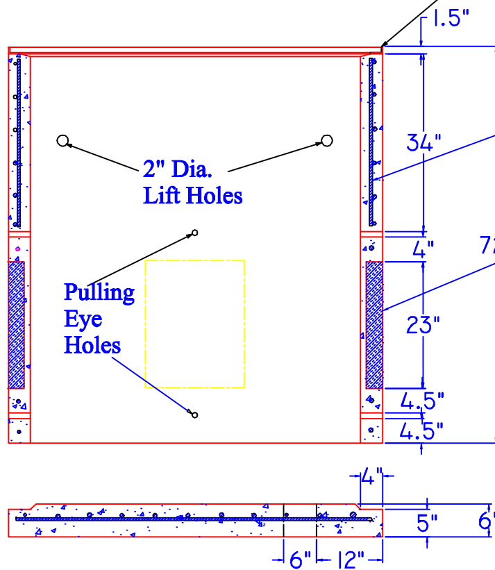
SECTION A-A
