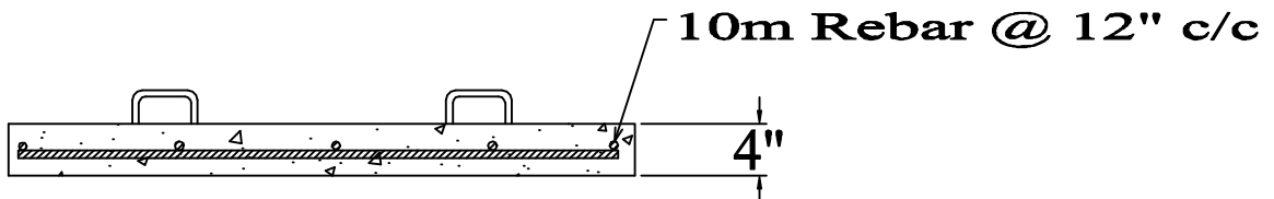
SECTION A-A
